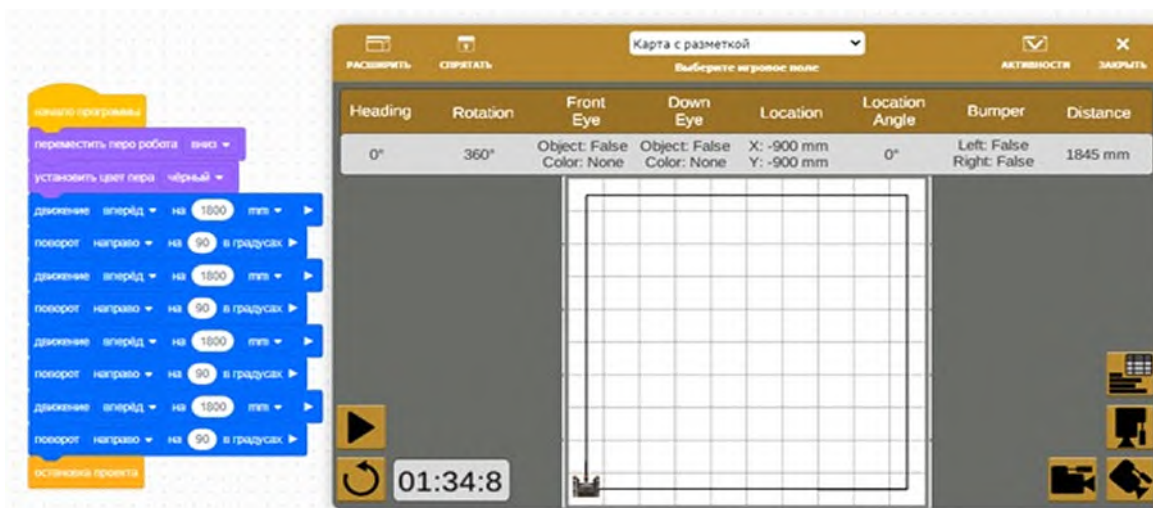
Рис. 12. Скрипт рисования роботом квадрата
