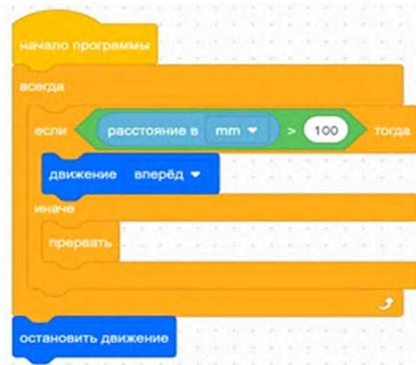
Рис. 31. Пример программы
