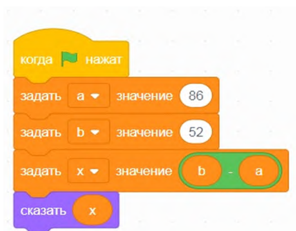
Рис. 118. Вид программы
