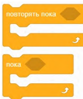
Рис. 25 — Блоки циклов
