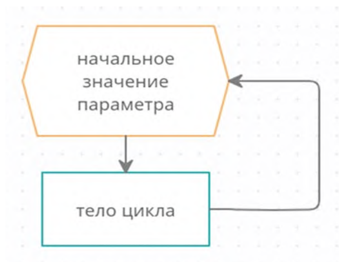
Рис. 124. Блок-схема цикла
