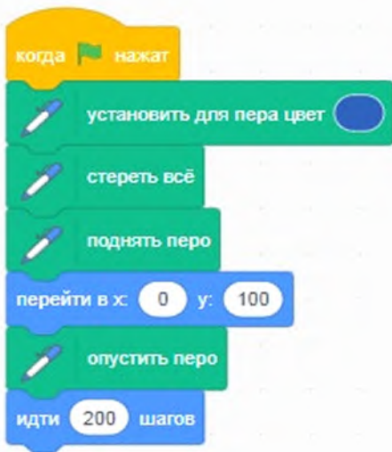
Рис. 103. Вид скрипта
