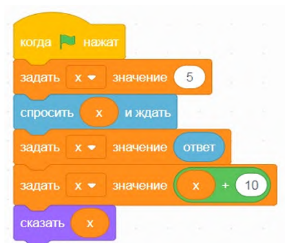
Рис. 117. Вид программы
